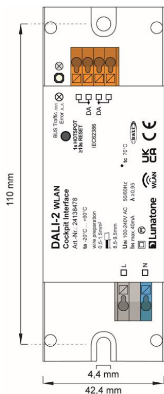
Abmessungen DALI-2 WLAN Cockpit Interface
