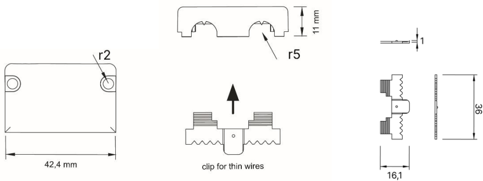
Standard Abdeckung Zugentlastung für 120x41x22mm
