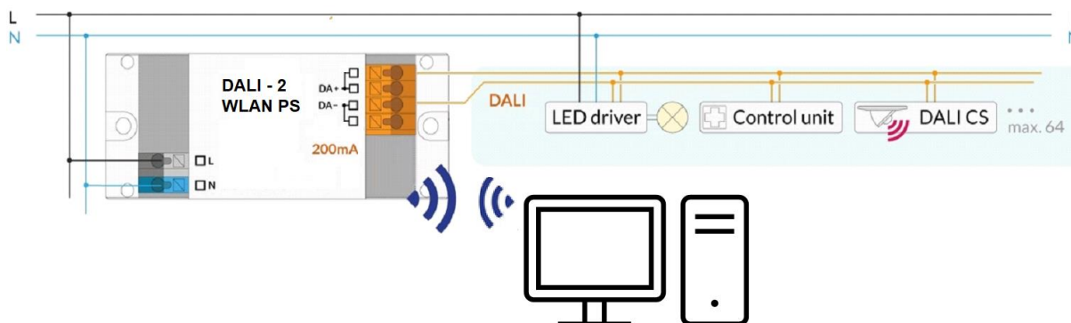
Abb. 1 Installation DALI-2 WLAN PS Cockpit Interface – typische Anwendung
