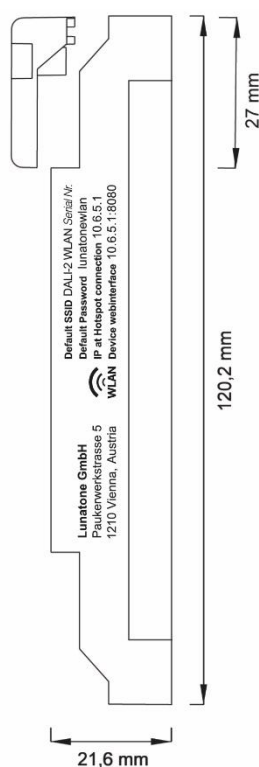
Abmessungen DALI-2 WLAN Cockpit Interface
