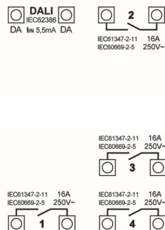
Anschlussplan 4x RM16 I HS
