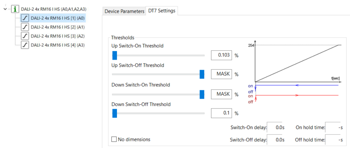
Abbildung 3 DALI Cockpit, 1. Relaiskontakt, Reiter: DT7 Einstellungen
