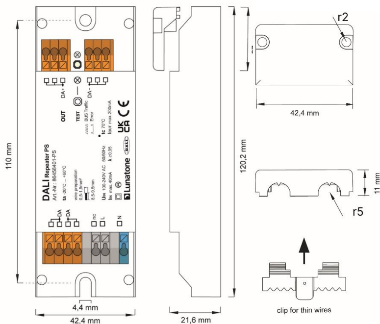
DALI Repeater PS Geometrie Deckeneinwurf Art. Nr. 86458401-PS
