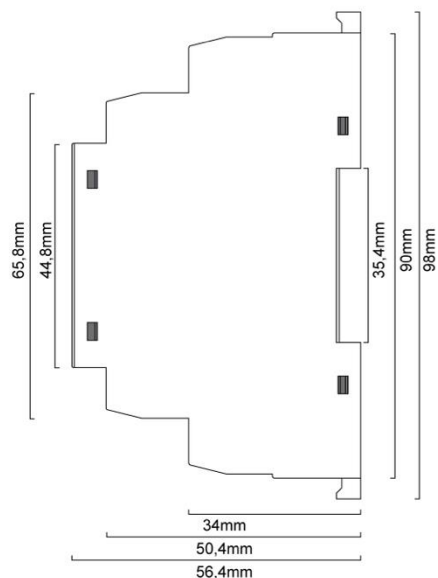
DALI Repeater Geometrie Hutschienenmodul Art Nr. 86458401
