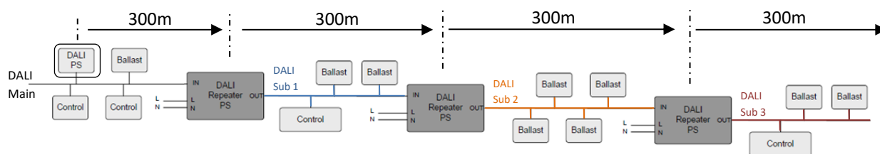
Abb. 2 Anwendungsbeispiel: Leitungslänge erhöhen
