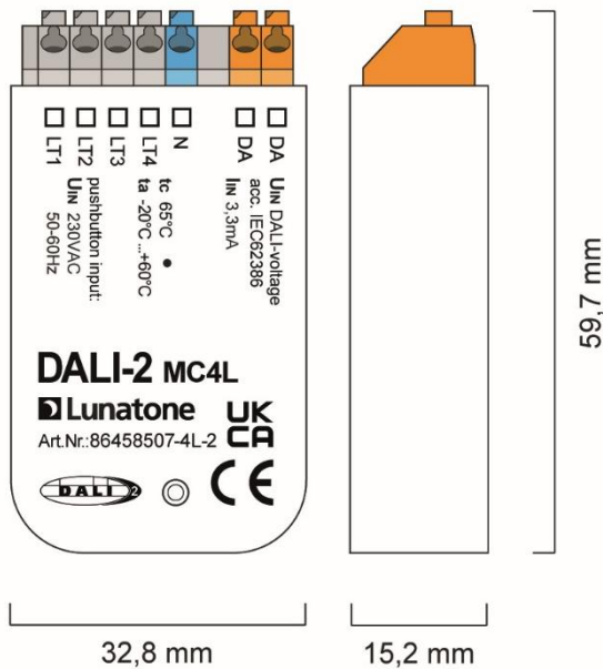
Abmessungen DALI-2 MC4L
