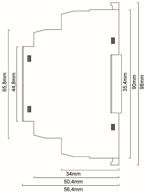
Abmessungen DALI-2 MC4L-HS
