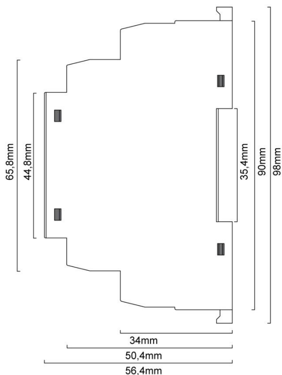
Abmessungen
